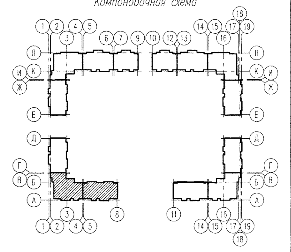
Компоновочная схема
